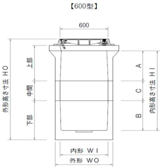
ハンドホール(一般型)サイズ表
