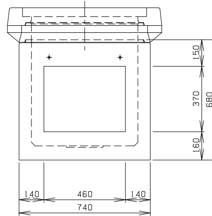
A 側 面 図
