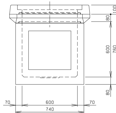
C 側 面 図
