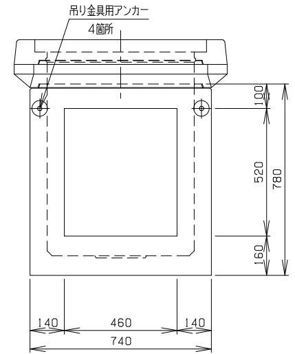
B 側 面 図
