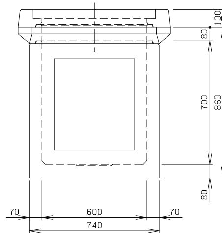
C 側 面 図
