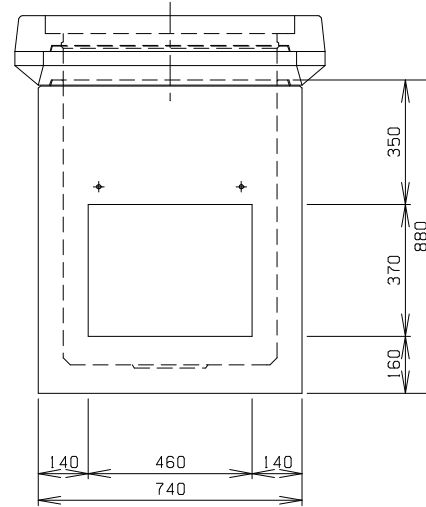
C 側 面 図
