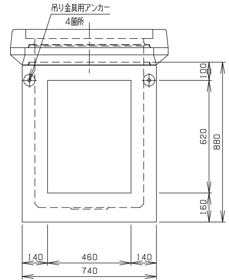
B 側 面 図
