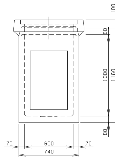
C 側 面 図
