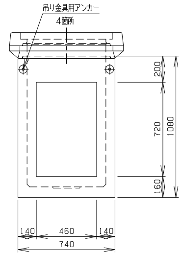
B 側 面 図
