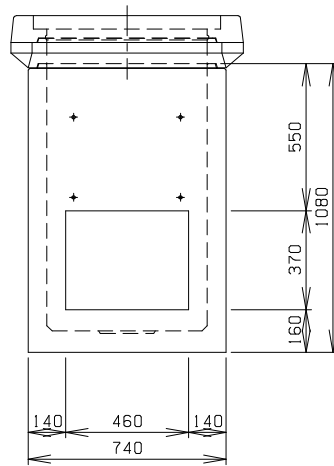
C 側 面 図
