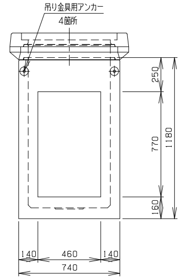
B 側 面 図
