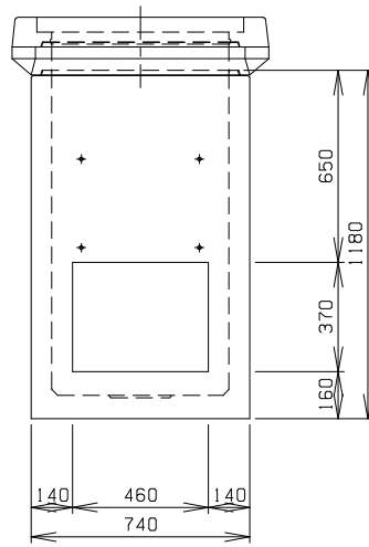
C 側 面 図
