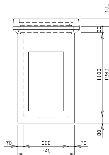
C 側 面 図
