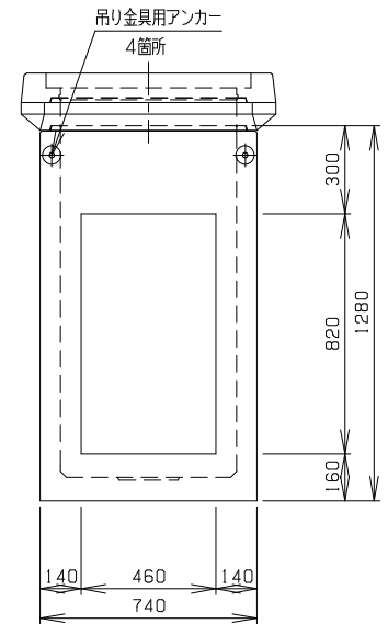
D 側 面 図
