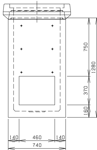
C 側 面 図
