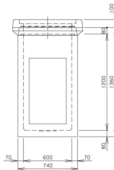
C 側 面 図
