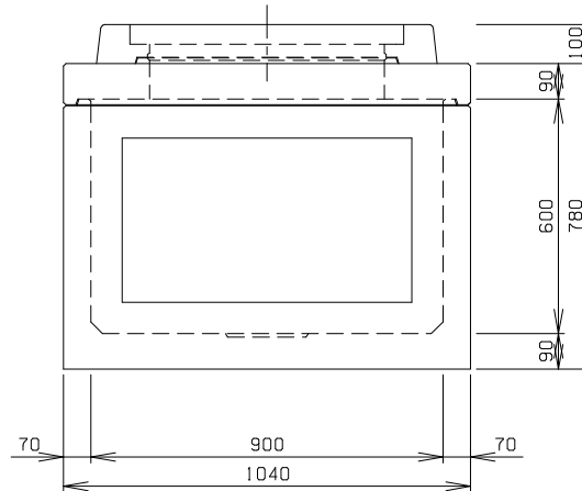
C 側 面 図
