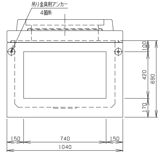
B 側 面 図
