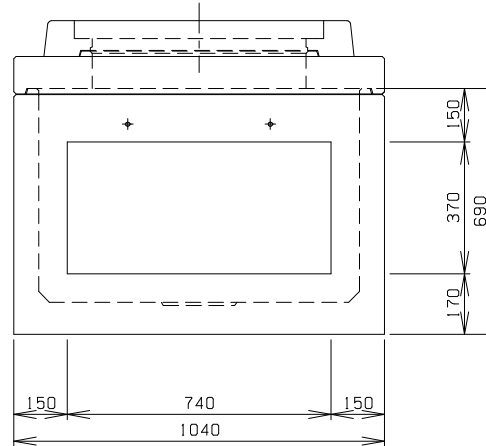
A 側 面 図
