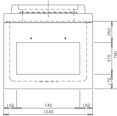
A 側 面 図
