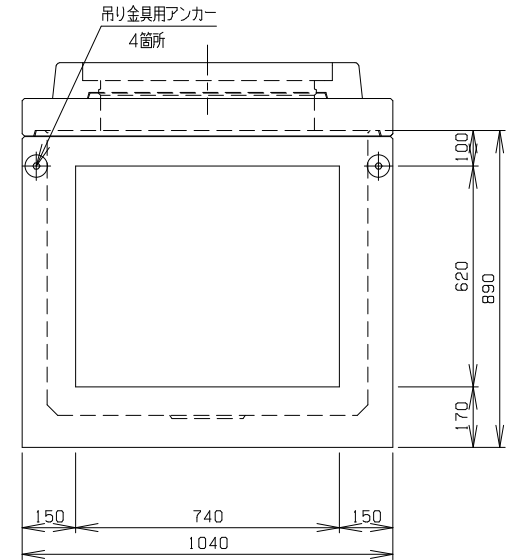
B 側 面 図
