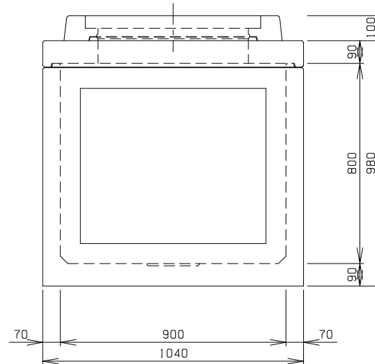
C 側 面 図
