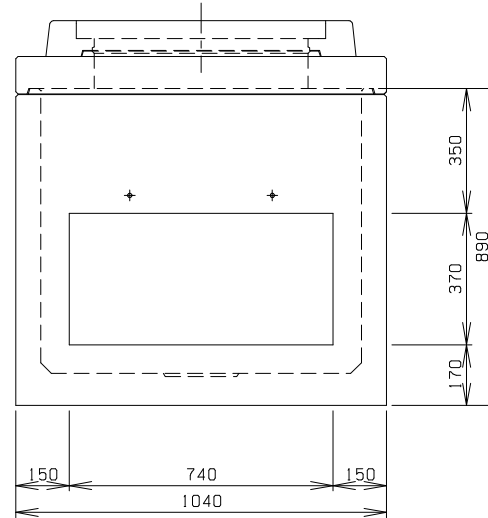
C 側 面 図
