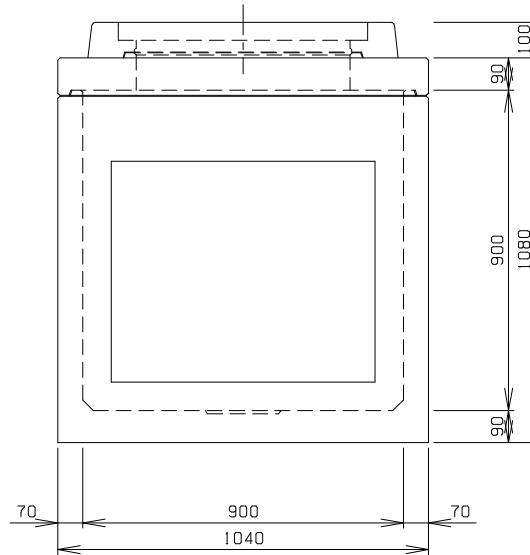
C 側 面 図
