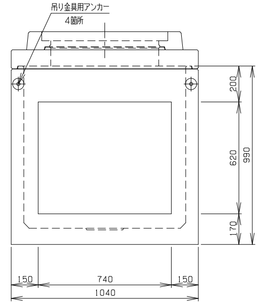
D 側 面 図
