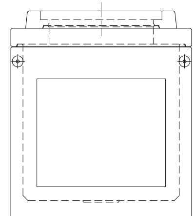
D 側 面 図
