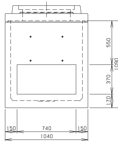
C 側 面 図
