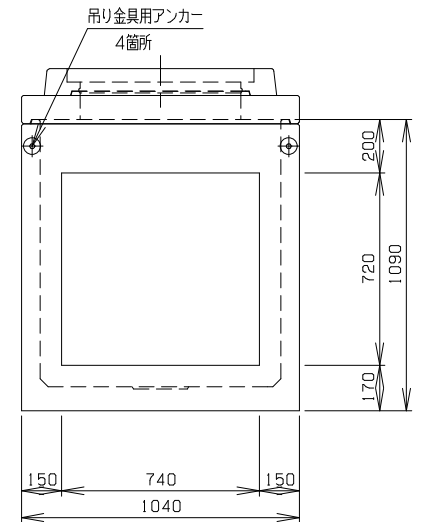
B 側 面 図
