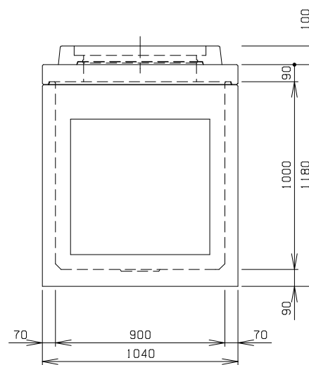
C 側 面 図
