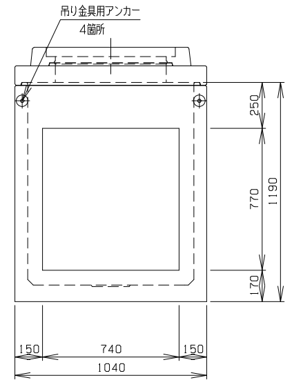
B 側 面 図
