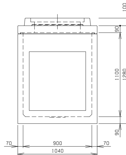
C 側 面 図
