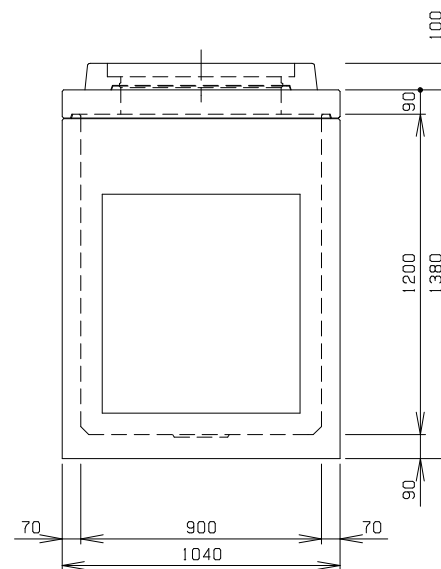
C 側 面 図
