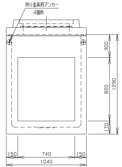
D 側 面 図
