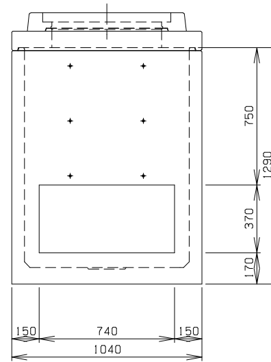
C 側 面 図
