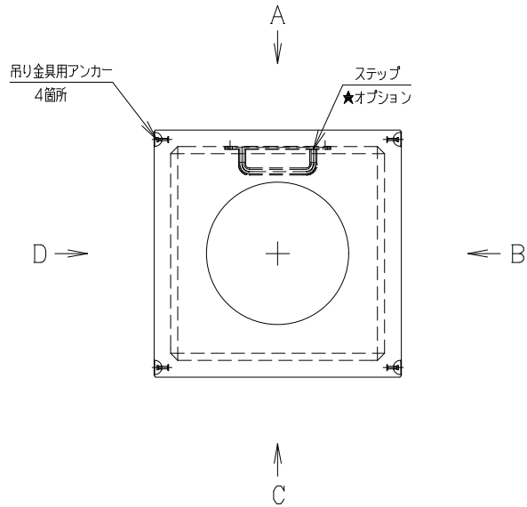
平 面 図
