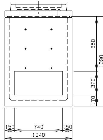
C 側 面 図
