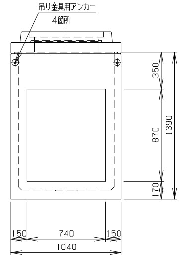
B 側 面 図
