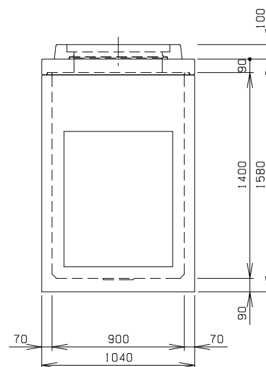
C 側 面 図
