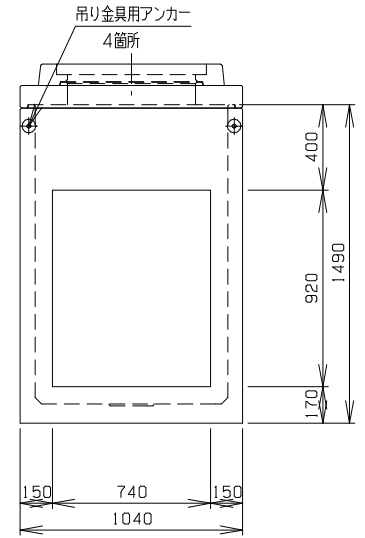
B 側 面 図
