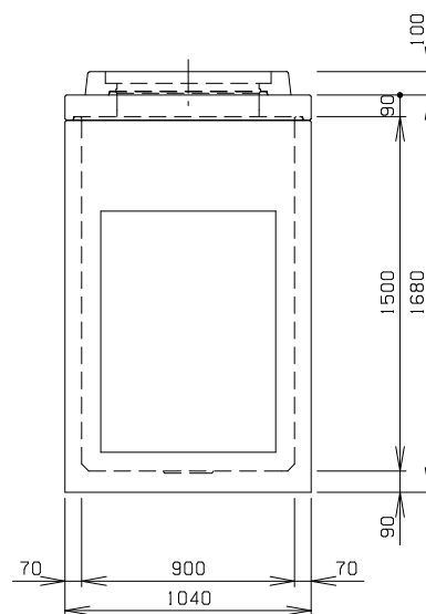
C 側 面 図
