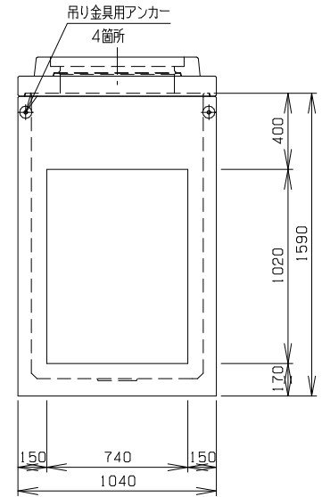
D 側 面 図
