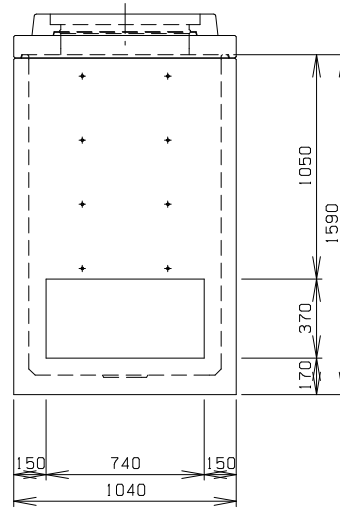
C 側 面 図
