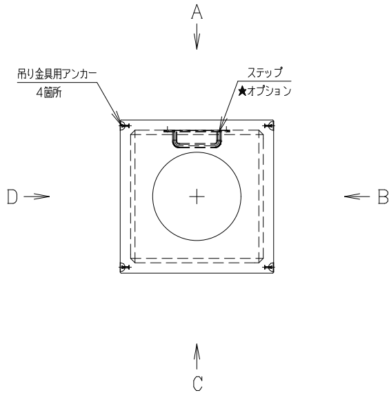
平 面 図
